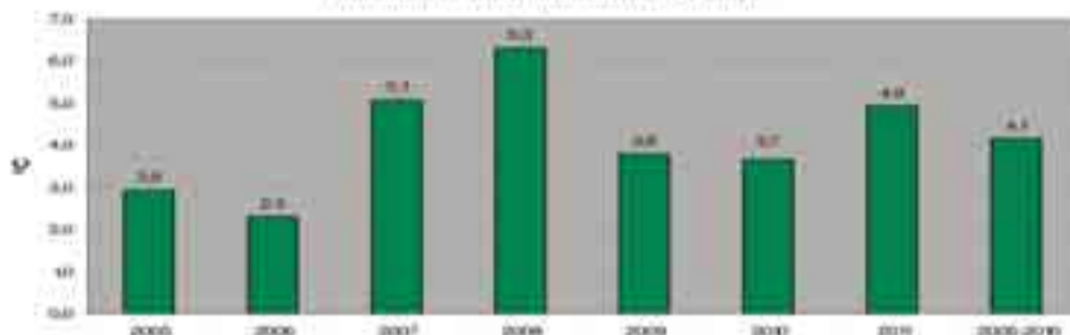
Observatori de Pujalt. Temperatura mitjana hiverna 2005-2011.
